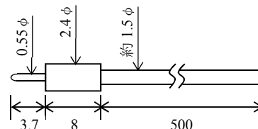
チェック用プラグ 外形図
