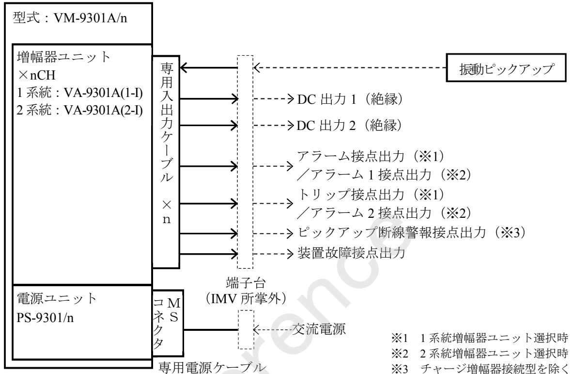
全体構成図 (ケーブル選択時)
