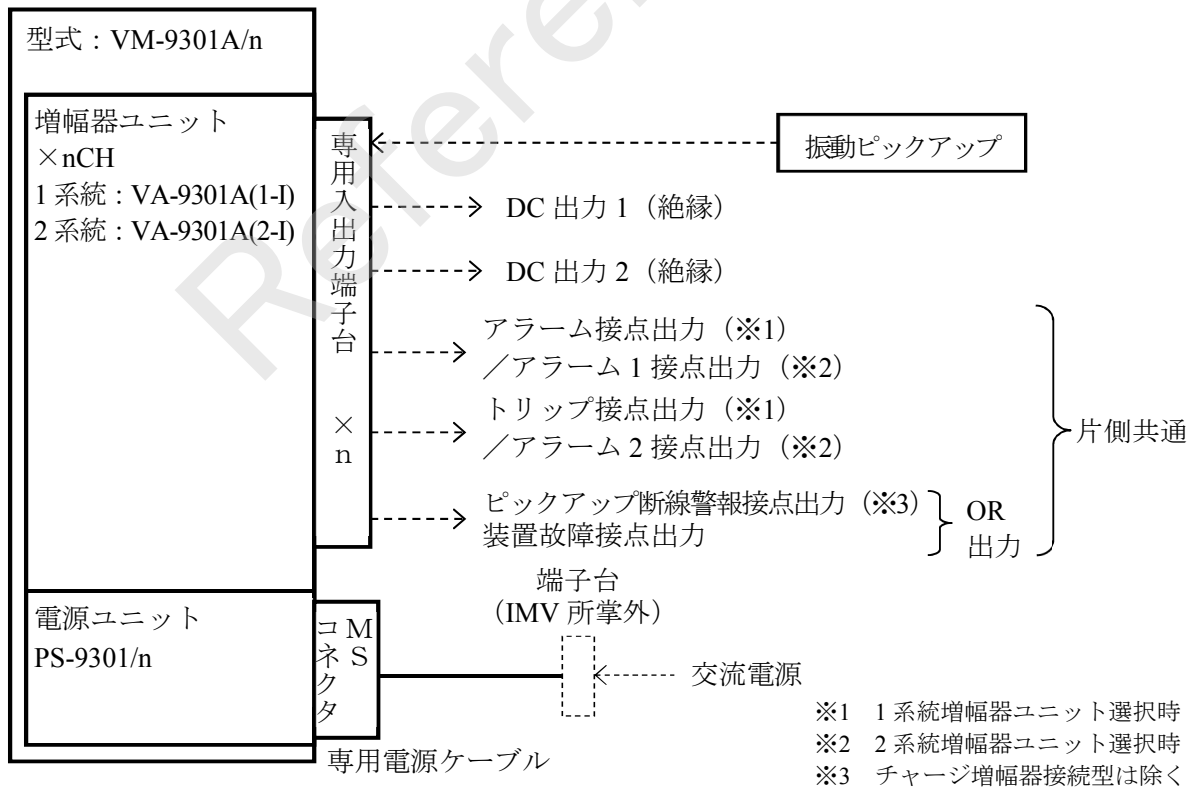
全体構成図（端子台選択時）
